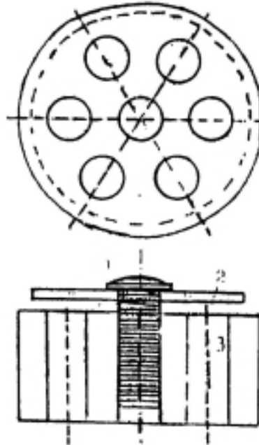
Gambar 3. Katup kaki
